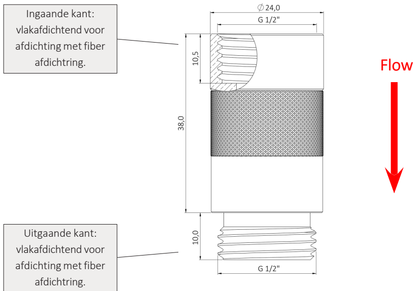
Afbeelding: Control Flow douche (afmetingen in mm)
